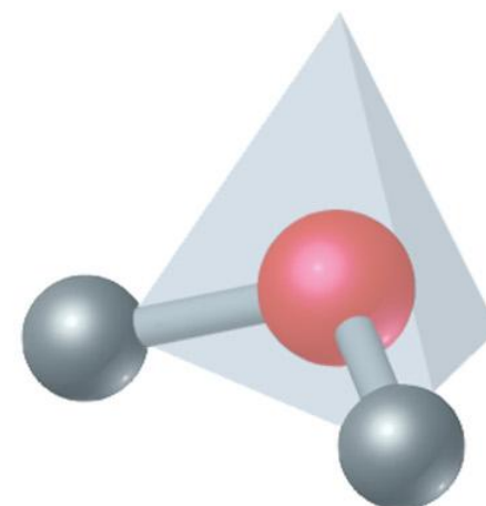
Bent
