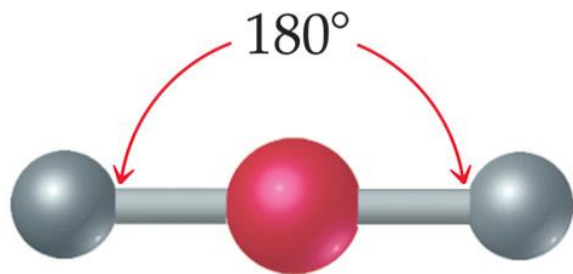
Linear
